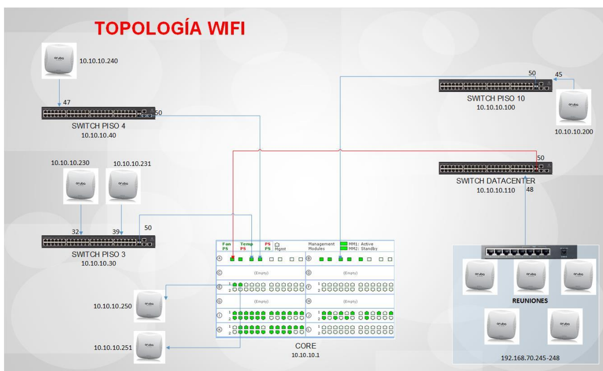
Ilustración 19 Topología WIFI
