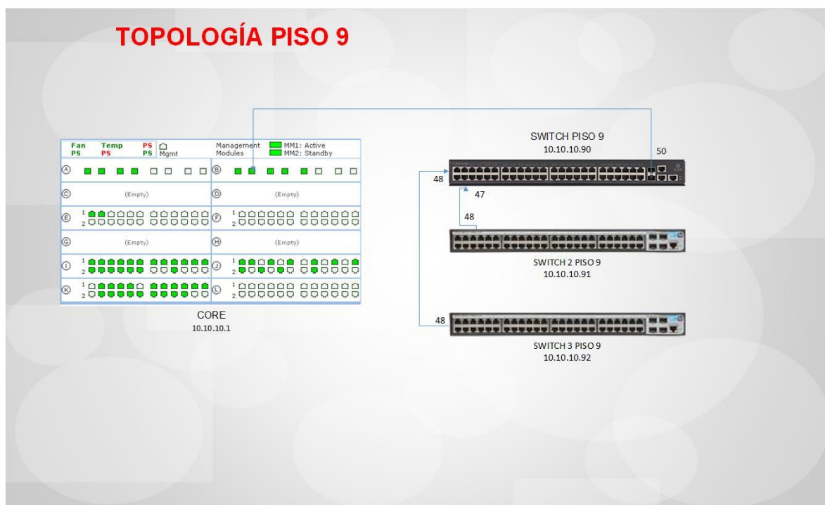
Ilustración 14 Conexión piso 9.
