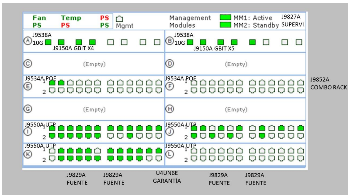
Ilustración 1 Equipo Core
