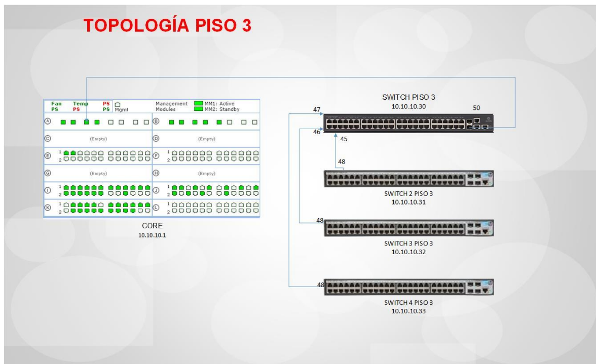
Ilustración 12 Conexión piso 3.
